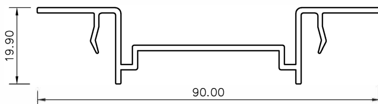
Perfil cerradero marco (hoja corredera)
