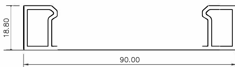
Perfil suplemento cerradero marco (hoja corredera)
