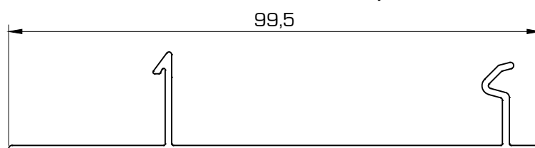
D0264 Lama celosía plana
