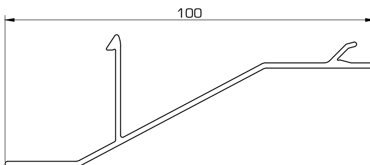
D0223 Lama celosía tipo "Z" recta
