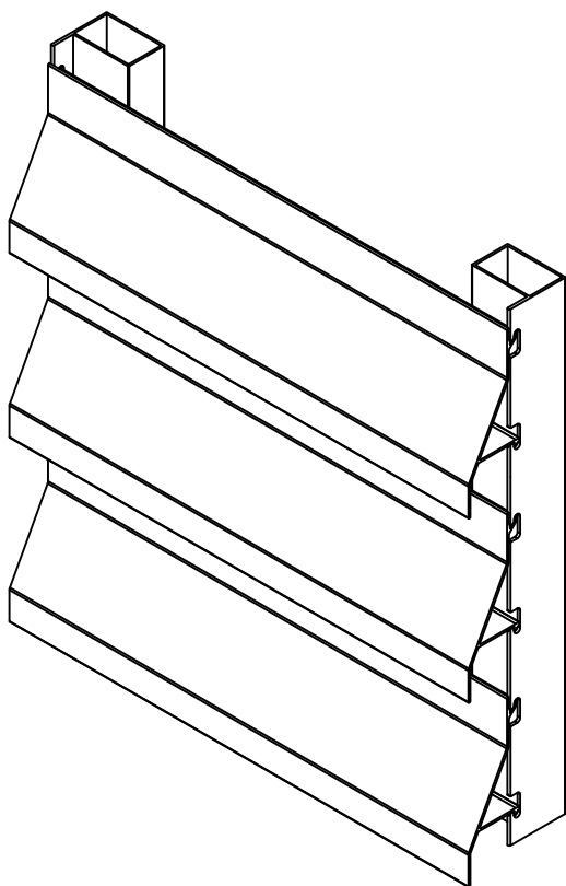
D0239 Lama celosía curva
