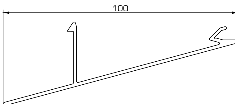
D0240 Lama celosía recta
