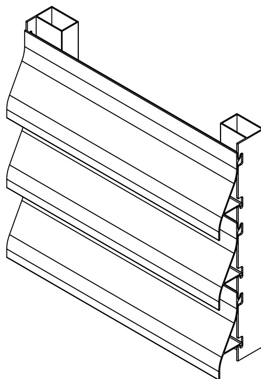
D0238 Lama celosía tipo "Z" curva
