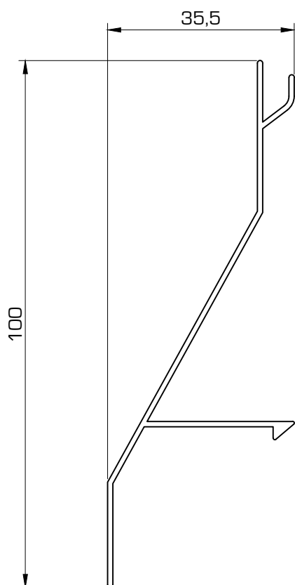
821 Lama ventilación para soporte 820
