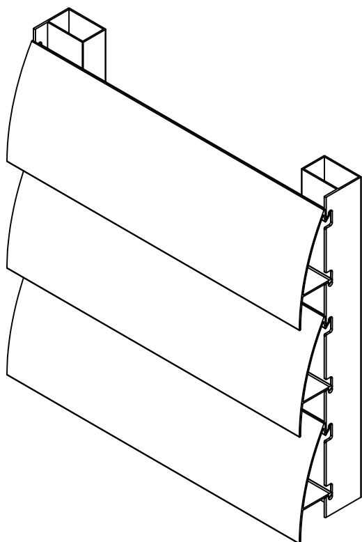
D0239 Lama celosía curva
