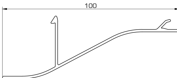
D0238 Lama celosía tipo "Z" curva
