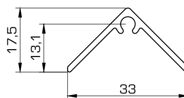
D0256 Angulo portatornillo
