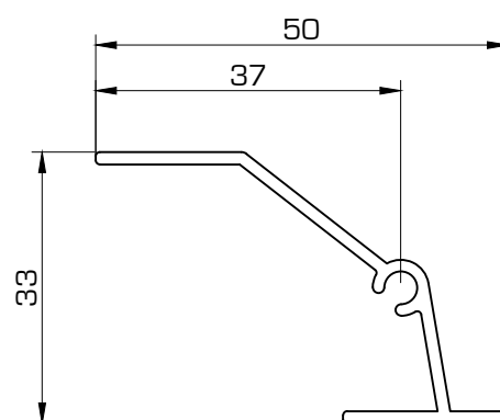
D0280 Celosía para atornillar
