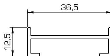
D0279 Soporte celosía
