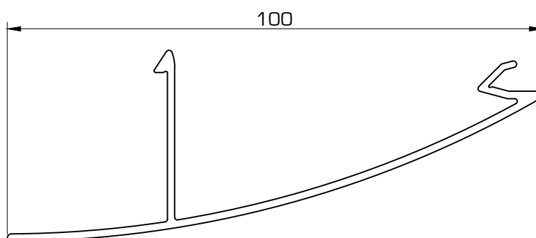
D0239 Lama celosía curva
