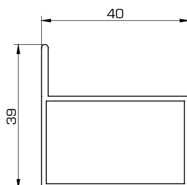
D0224 Soporte celosía
