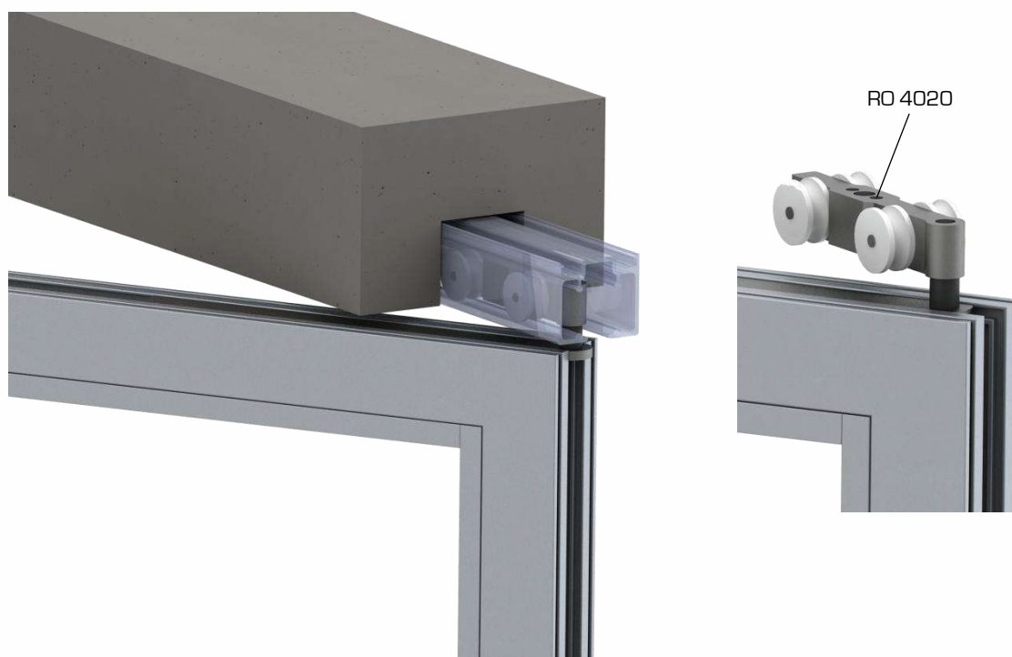
Guía superior encastrada – Rodamiento Superior Hojas Pares
