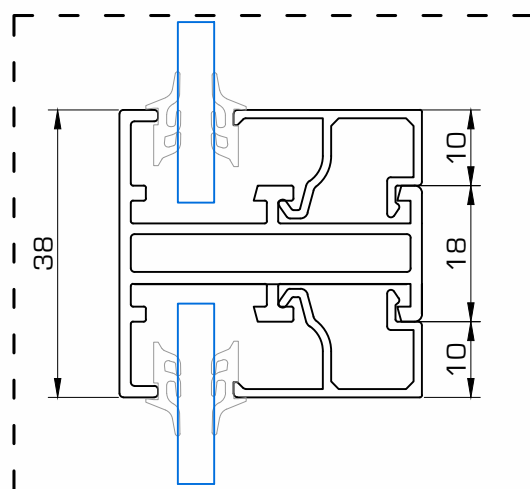
Detalle con junquillo
