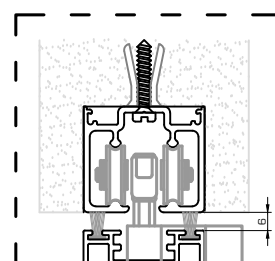
Detalle guía embutida
