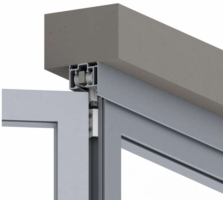
Guía superior con ala – Bisagra Tandem superior
