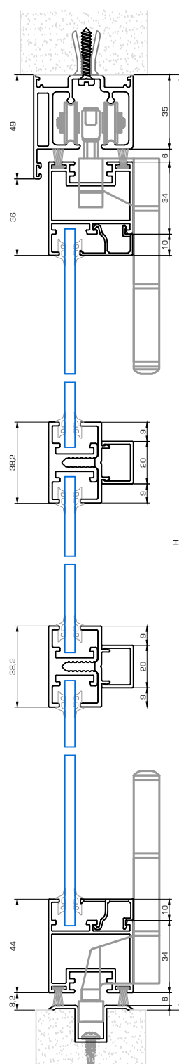
Detalle guía embutida
