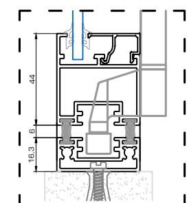
Detalle marco inferior
