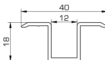
487 Guía inferior empotrada
