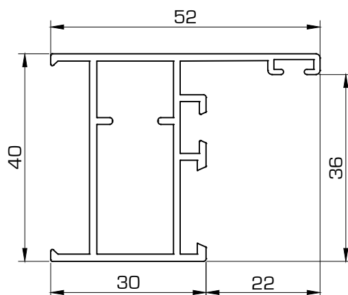
5400 Marco de 40 x 52
