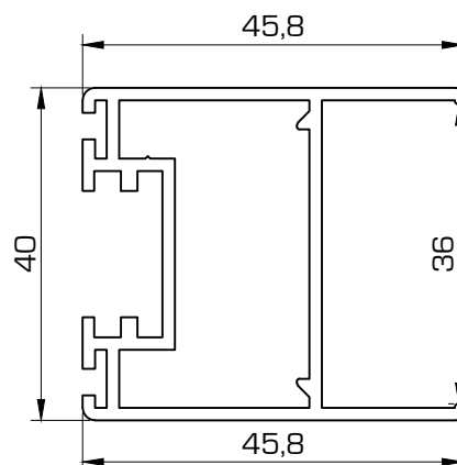
4705 Hoja plegale mallorquina
