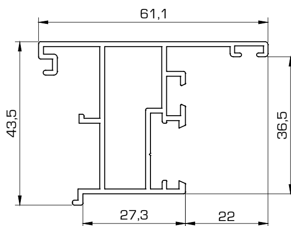
5402 Perfil inversor
