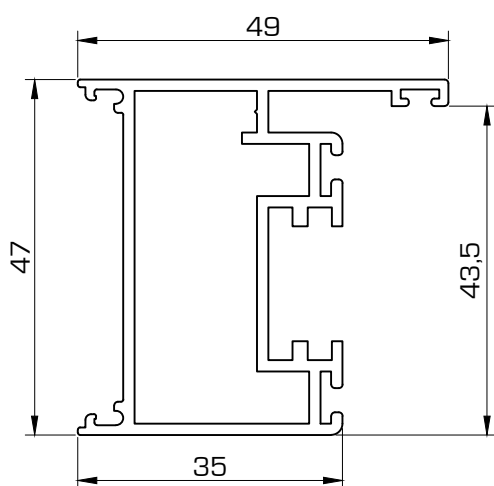
482 Marco lateral e inferior
