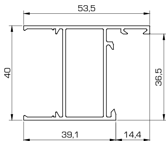
450 Hoja mallorquina 40 x 20
