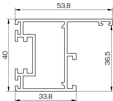
484 Hoja plegable europea
