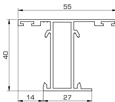
458 Travesaño 40 x 20
