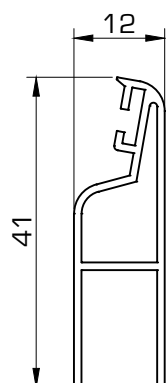
454 Lama fija 57,5 453 Lama fija 41 457 Lama ovalada
