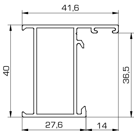
400 Marco 40 x 20
