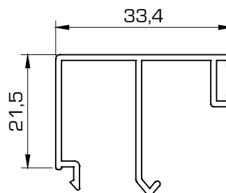
1406 Junquillo recto 33 mm
