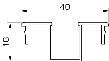
455 Guía compensación 456 Lama móvil
