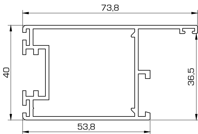
485 Hoja plegable puerta
