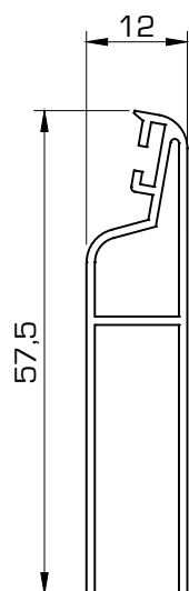
454 Lama fija 57,5 453 Lama fija 41 457 Lama ovalada
