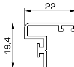
472 Perfil batiente
