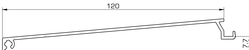
D0174 Alargadera 120 mm
