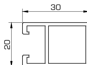
651 División muebles una salida 30 x 20 mm
