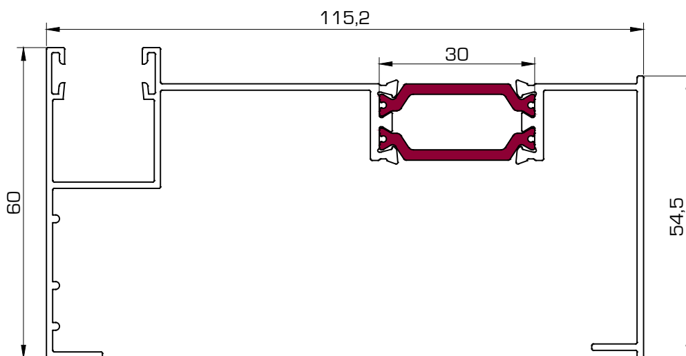
203 Guía compacto de 110 mm
