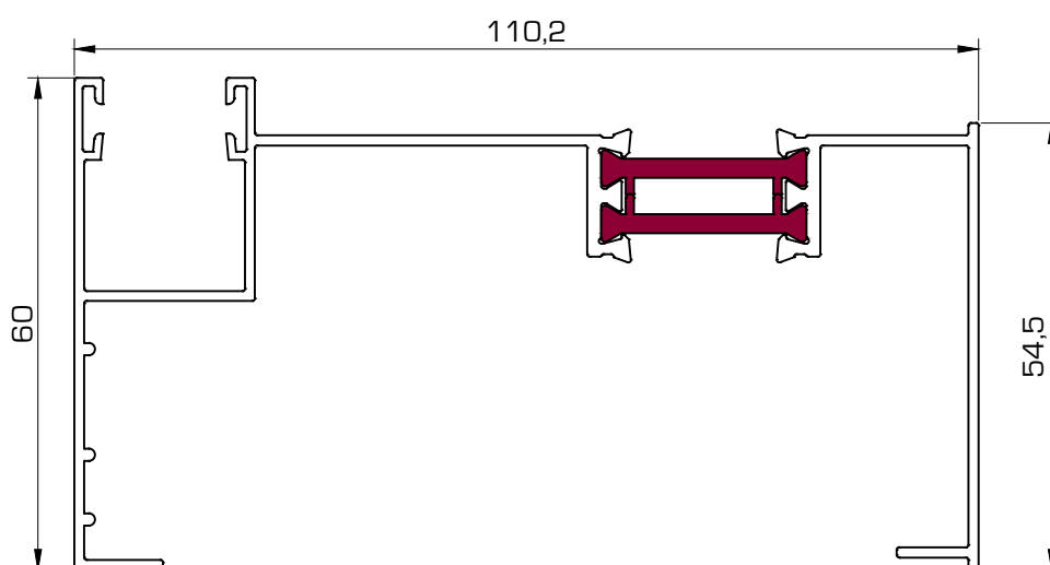
208 Guía compacto de 100 mm
