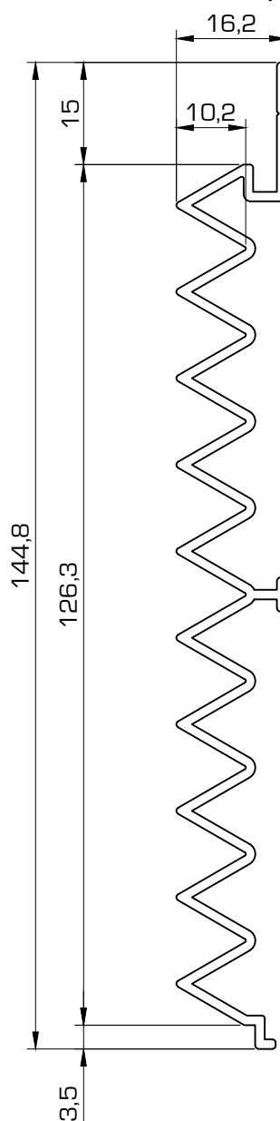
D5991 Lama onda picos 10,2 mm
