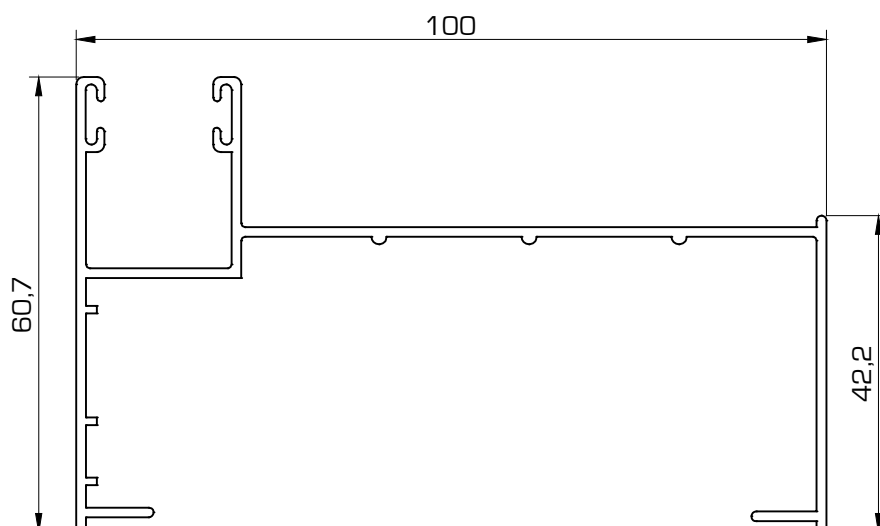
214 Guía compacto de 100 mm
