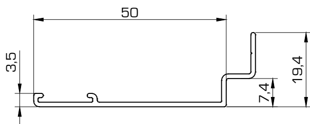
5053 Tapajuntas marco 50 mm
