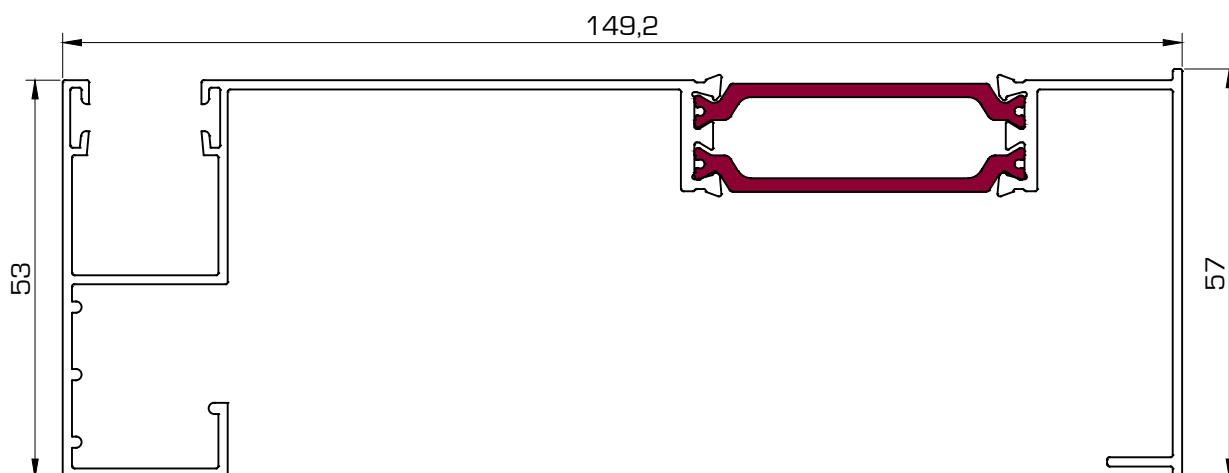
211 Guía compacto de 150 mm
