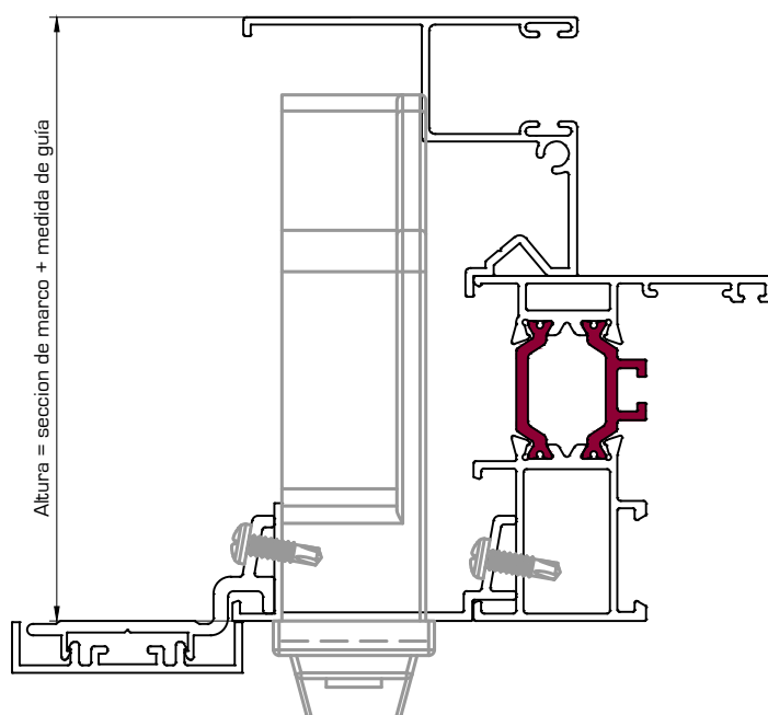
DETALLE COLOCACIÓN GUÍAS EXTERIORES CON ACLOPE 224 Y SOLAPE 5030
