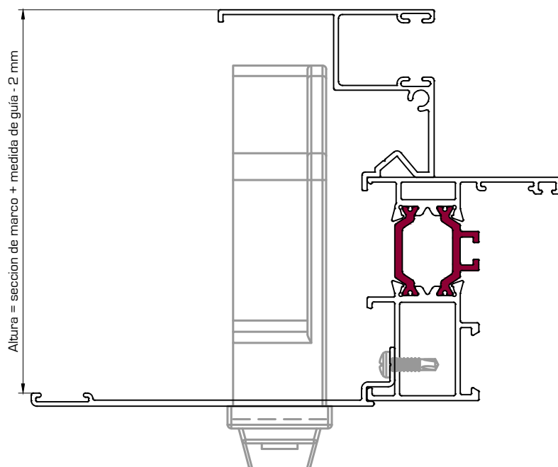
DETALLE COLOCACIÓN GUÍAS EXTERIORES CON SOLAPE 5059
