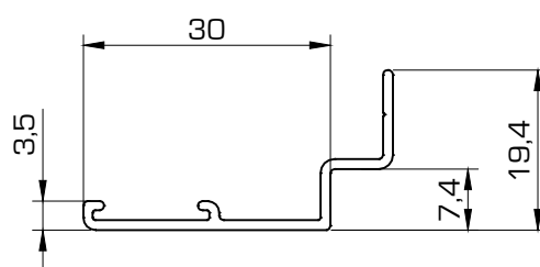
5033 Tapajuntas marco 30 mm
