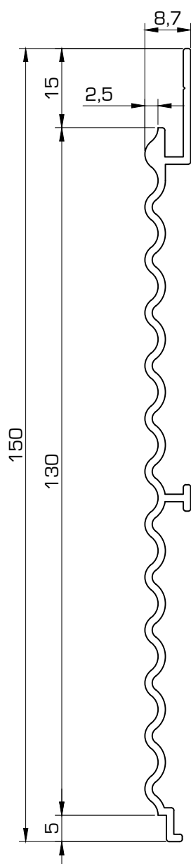
D5816 Lama onda 2,5 mm
