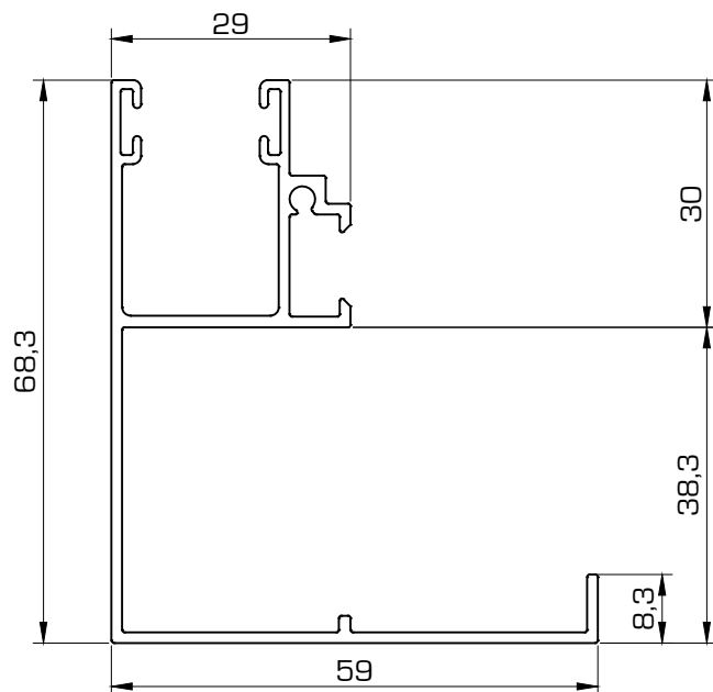
234 Guía marco puerta clip
