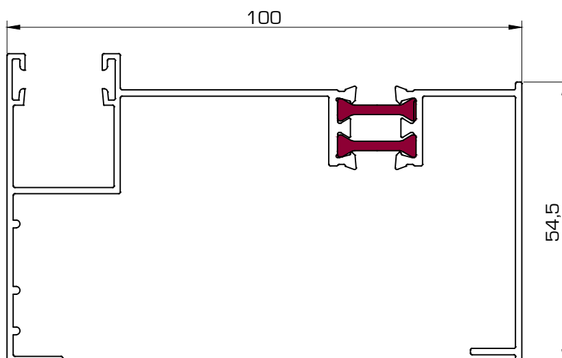
208 Guía compacto de 100 mm
