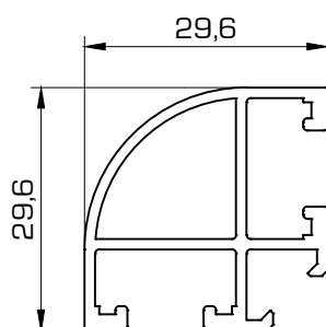
650 Esquinero muebles 30 x 30 mm
