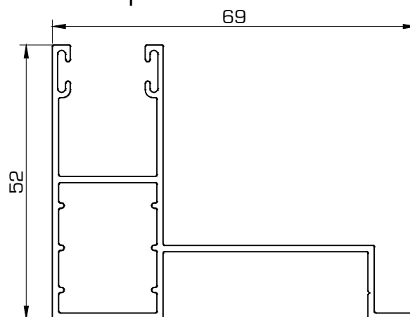
209 Guía para motor 60 mm
