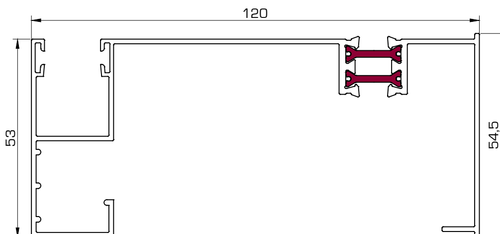
216 Guía compacto de 120 mm
