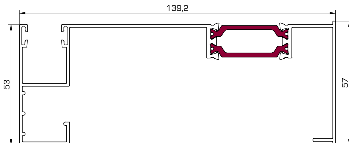
210 Guía compacto de 140 mm
