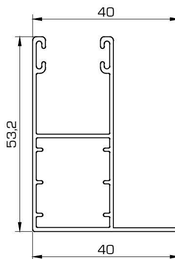
239 Guía con ala
