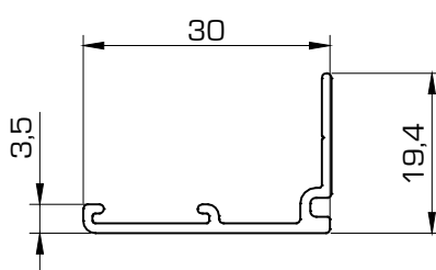
5034 Tapajuntas guía 30 mm
