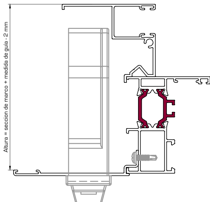
DETALLE COLOCACIÓN GUÍAS EXTERIORES CON SOLAPE 5057
