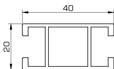
652 División muebles dos salidas 40 x 20 mm
