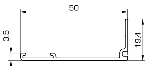
5054 Tapajuntas guía 50 mm
