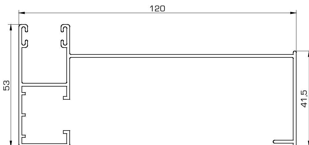
215 Guía compacto de 120 mm
