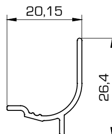
4605 Perfil vierteaguas
