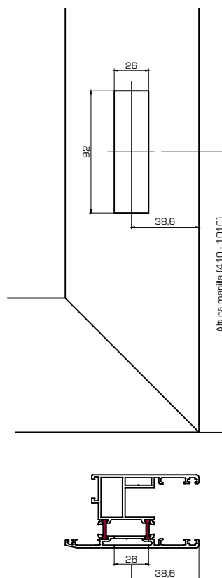
Mecanizado tirador uñero exterior.
