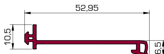
U066 Goma encuentro cruce P.V.C.
