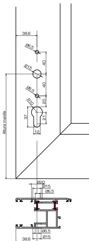
Mecanizado manilla int. y ext. con PZ
