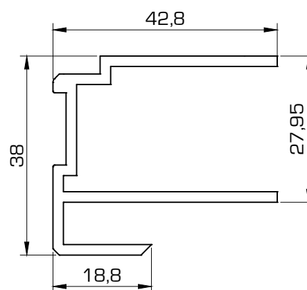
4607 Unión 4 hojas
