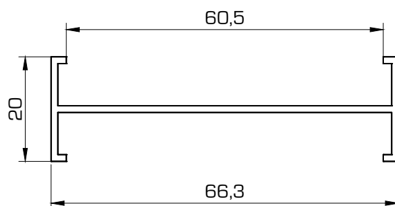
310 Unión de marcos
