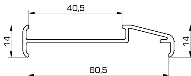
311 Unión abatible corredera
