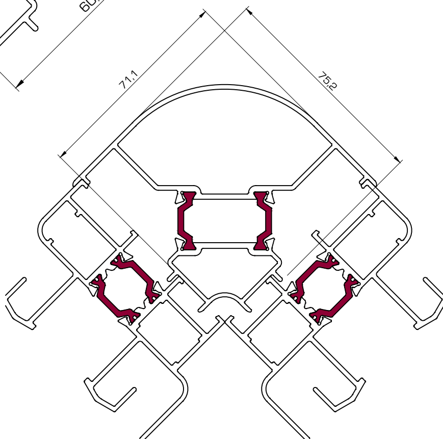
Detalle montaje esquinero 90º
