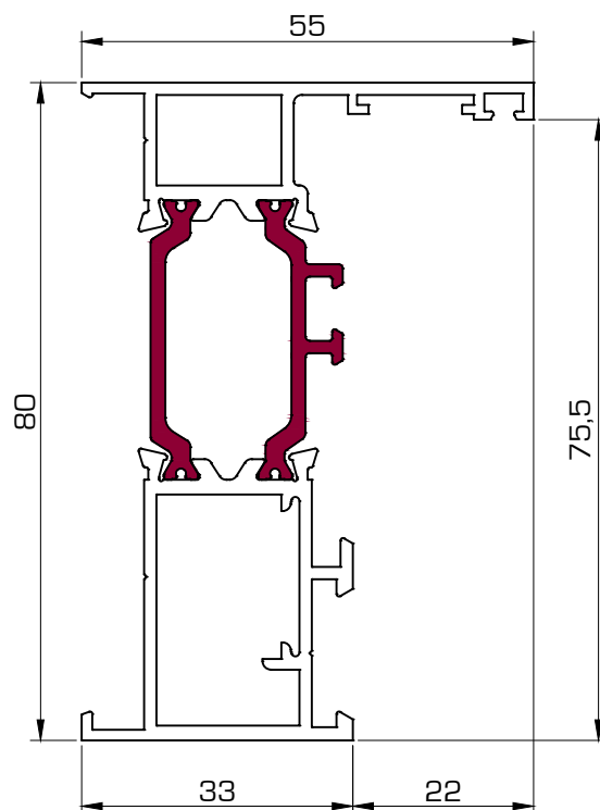
6000 Marco ventana
