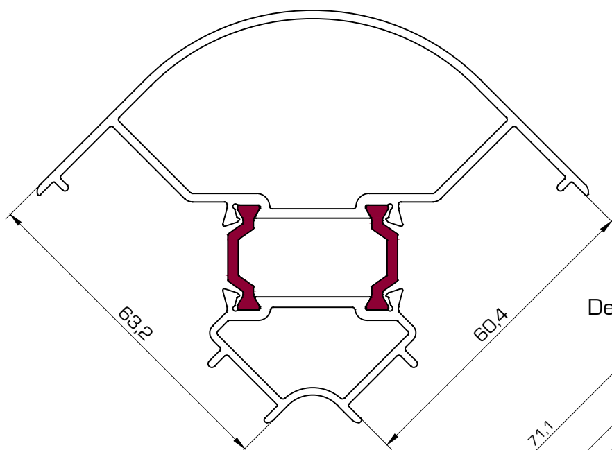
5008 Esquinero 90º
