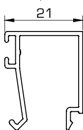
1414 Junquillo 21 mm
