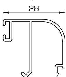
1436 Junquillo 28 mm
