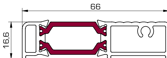
5940 Solera 66 mm
