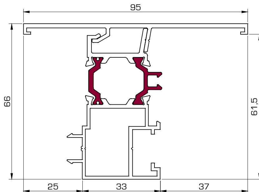
5952 Inversor H.O.
