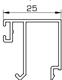
5013 Junquillo 25 mm
