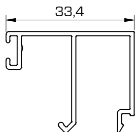
1406 Junquillo 33 mm
