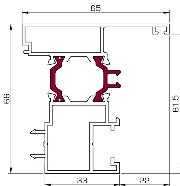
5902 Inversor
