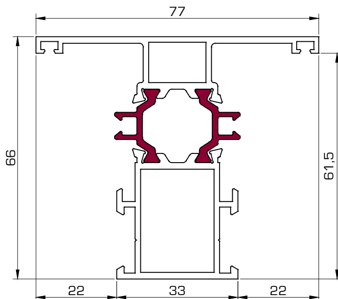
5904 Travesaño 33 mm
