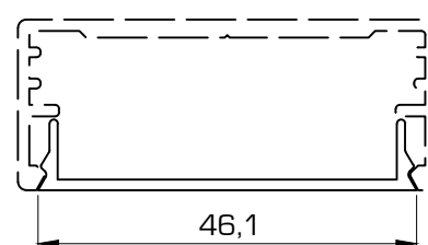
D3504 Tapa anclaje
