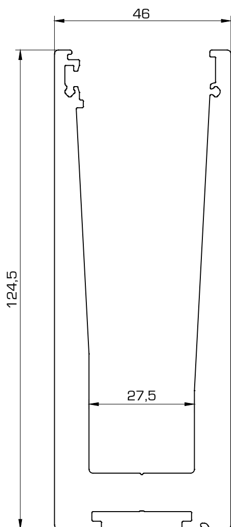
640 Perfil en U
