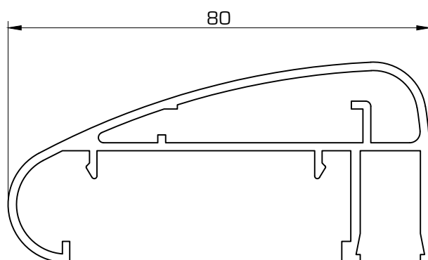
D3506 Pasamanos ovalado para vidrio
