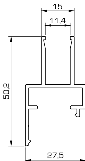
D3507 Perfil para vidrio completo
