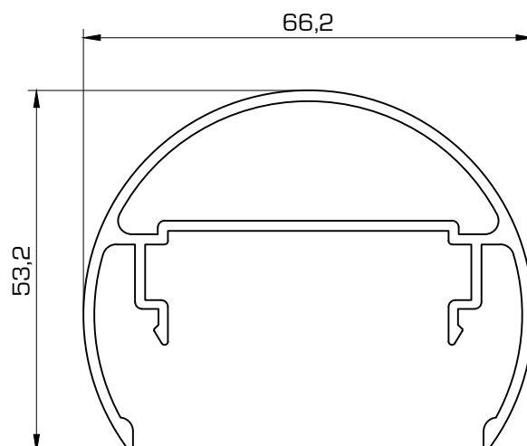
D3501 Pasamanos redondo
