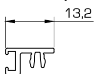
D3543 Clip fijo
