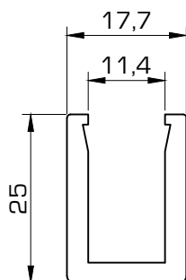
D3510 Remate vidrio
