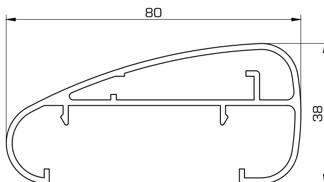
D3509 Pasamanos elíptico.
