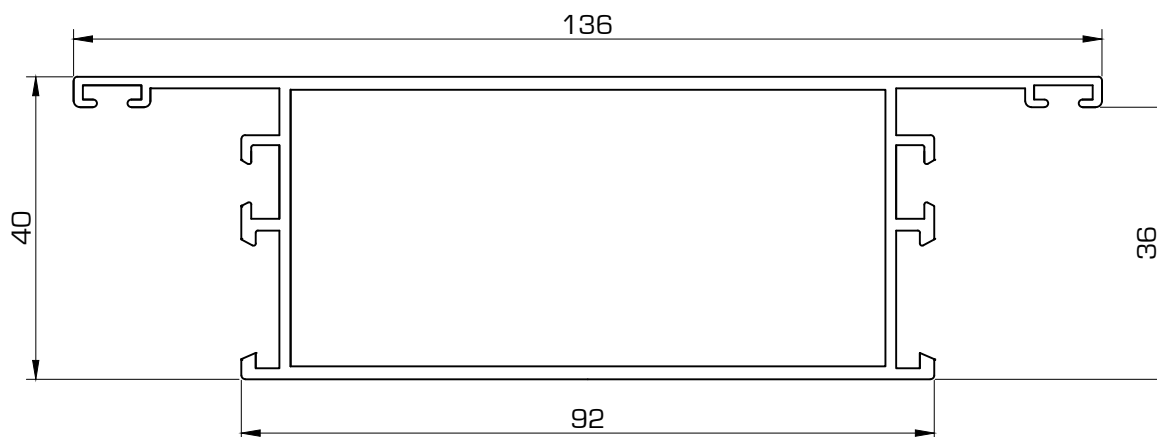
1425 Zócalo central
