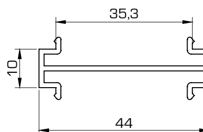
436 Perfil unión
