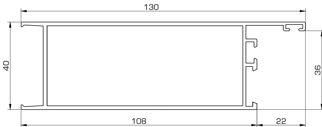
1426 Zócalo inferior
