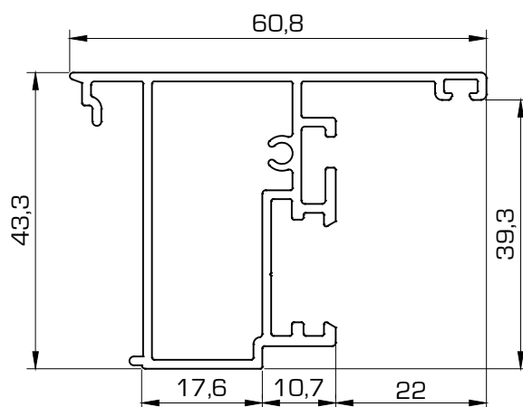
5402 Inversor
